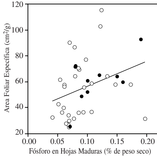
Fig. 3. Relación entre la concentración de fósforo en hojas maduras y su área foliar específica (Spearman r = 0.5498 ; p < 0.001 ). \circ = Datos de Cavalier 1986; \bullet = Datos del presente estudio.
