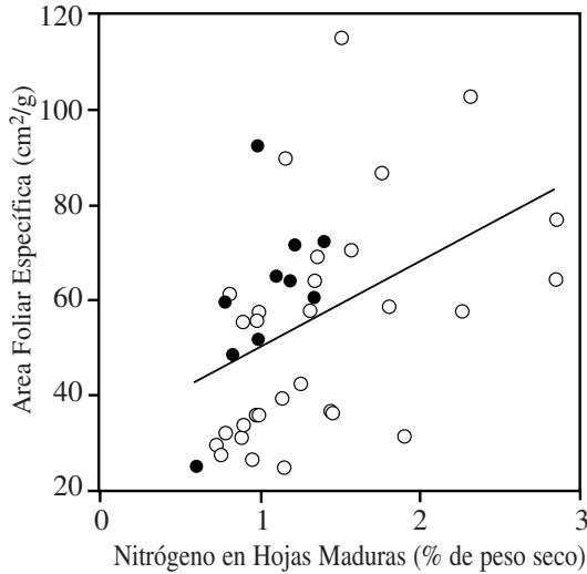
Fig. 2. Relación entre la concentración de nitrógeno en hojas maduras y su área foliar específica (Spearman r = 0.5498 ; p < 0.001 ). \circ = Datos de Cavalier 1986; \bullet = Datos del presente estudio.
